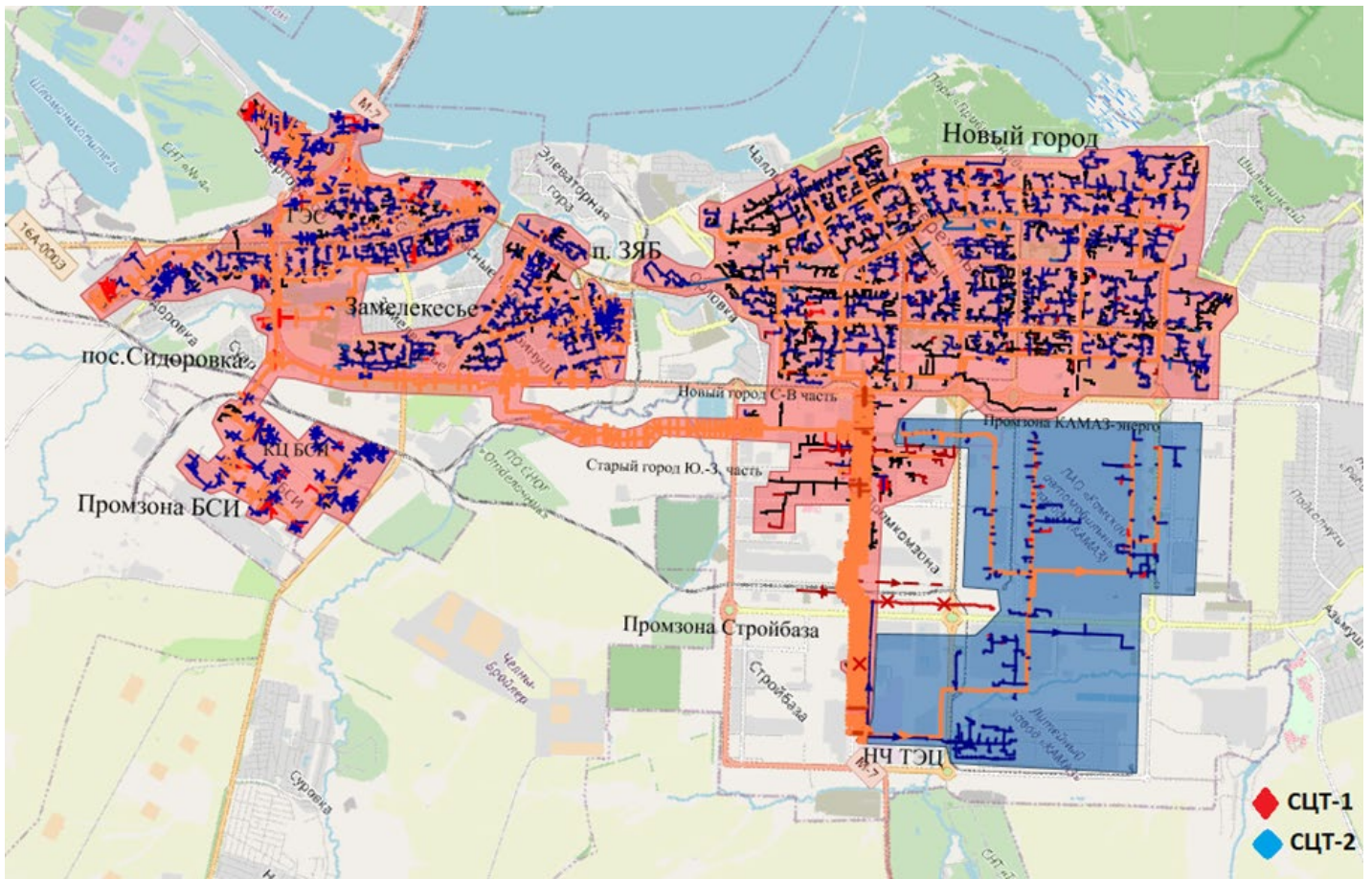
Рис.1 1. Зоны действия централизованных систем теплоснабжения города Набережные Челны
